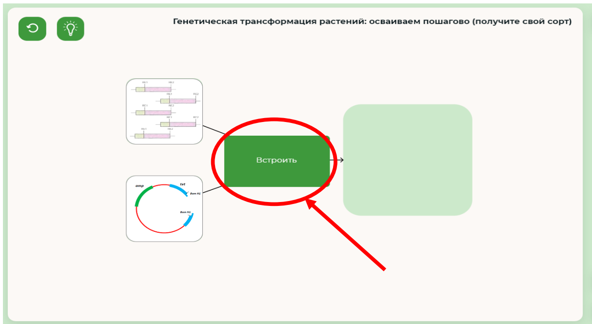
Рис. 5. Встраивание гена
